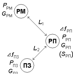
Рис. 1. РМ — радиомикрофон; РП — радиоприёмник; ПЗ — постановщик помех.
